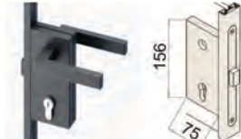
⑪ CERRADURA VERTICAL MAGNÉTICA CON LLAVE
